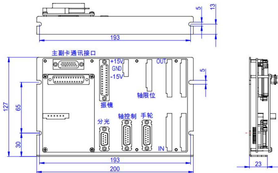
PCIE 端子板
