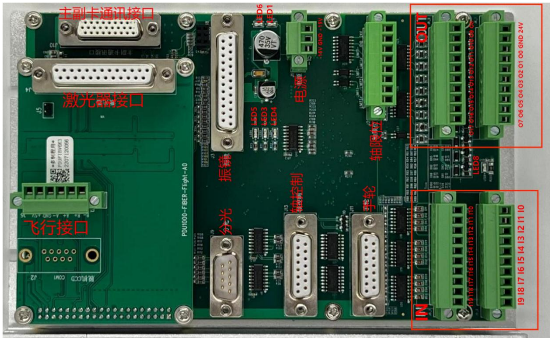
PCIE 端子板
